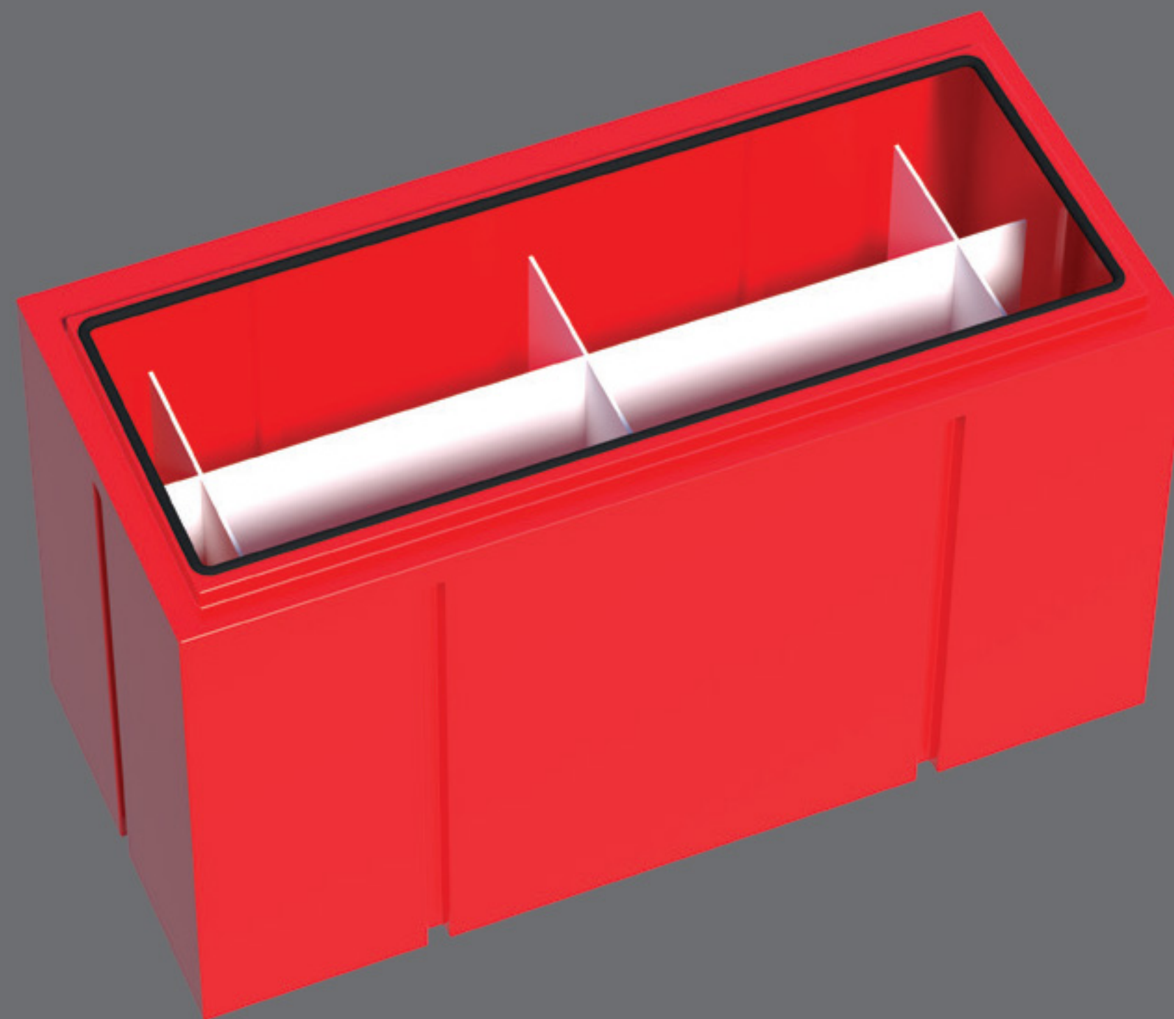
ถังบรรจุน้ำไม่น้อยกว่า 700 ลิตร ผลิตจากไฟเบอร์กลาส Fiberglass Reinforced Plastic (FRP.) ภายในถังเสริมแผ่นกั้นกระแทก (Baffle Plate) กันเป็นช่อง
