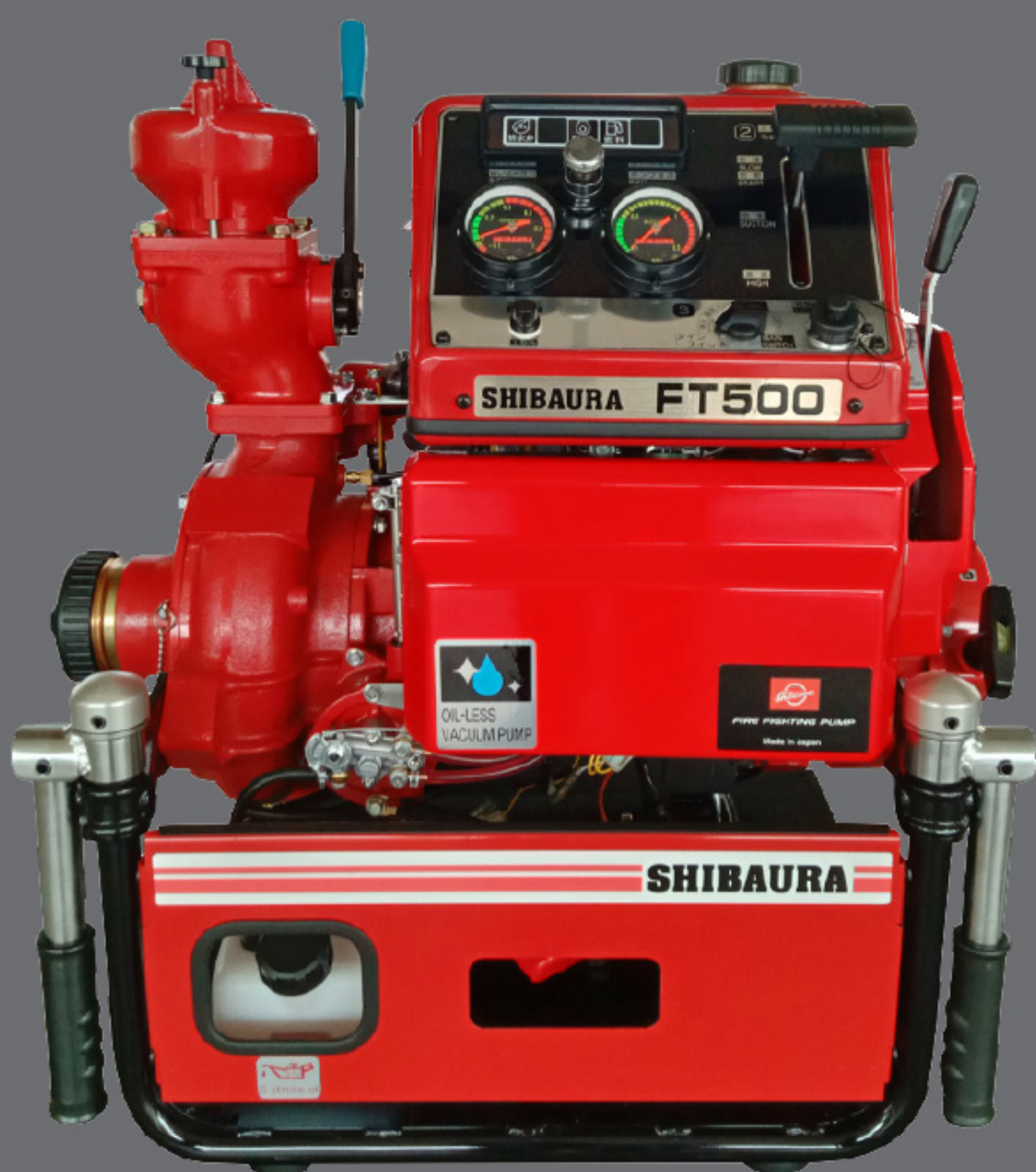
เครื่องสูบน้ำหยาบเบาเบนซิน 1450 ลิตร/นาที
